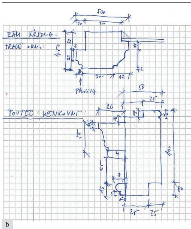
Praha, městská část Malá Strana, Hrzánský palác čp. 490/III, Velkopřevorské náměstí: a – terénní skica členění okna s profilací stojky rámu vnitřního okna; b – profilace venkovního poutce, vnitřního přičínku, klapaček a rámu vnitřního okenního křídla (D. Havlíková).
