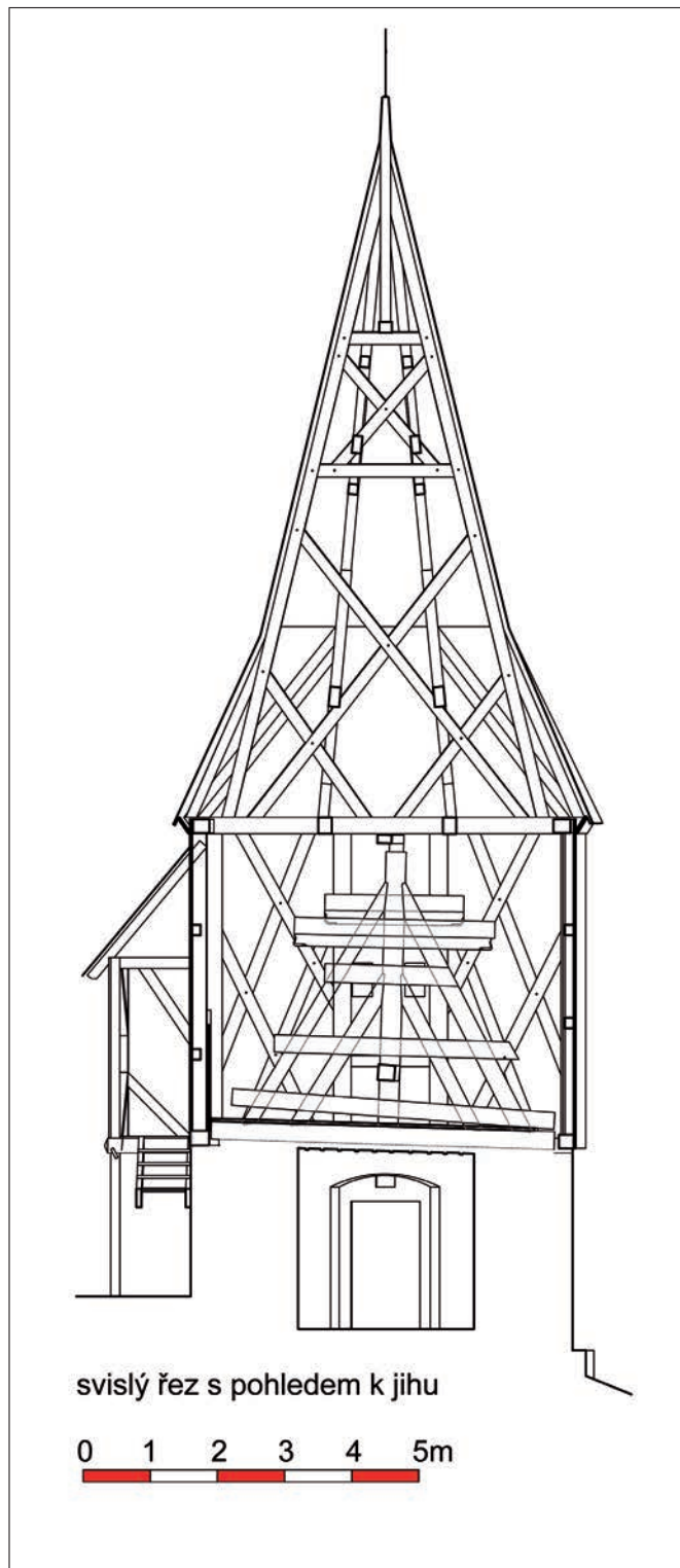
Vitice (okres Kolín), zvonice u kostela sv. Šimona a Judy, svislý řez (zaměření J. Veselý, J. Kypta).
