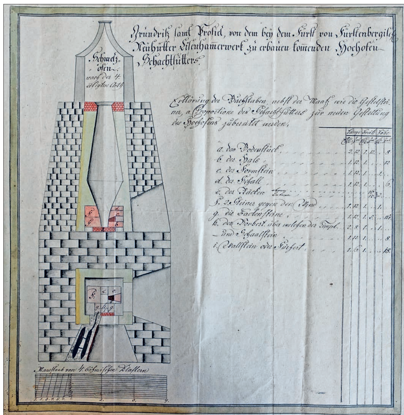
Nížbor (okres Beroun), Plán na výstavbu vysoké pece v Nové Huti z roku 1810 (SOA Praha, Vs Křivoklát, Ústřední správa, inv. č. 189, sig.US-55-1-11, kart. 14)
