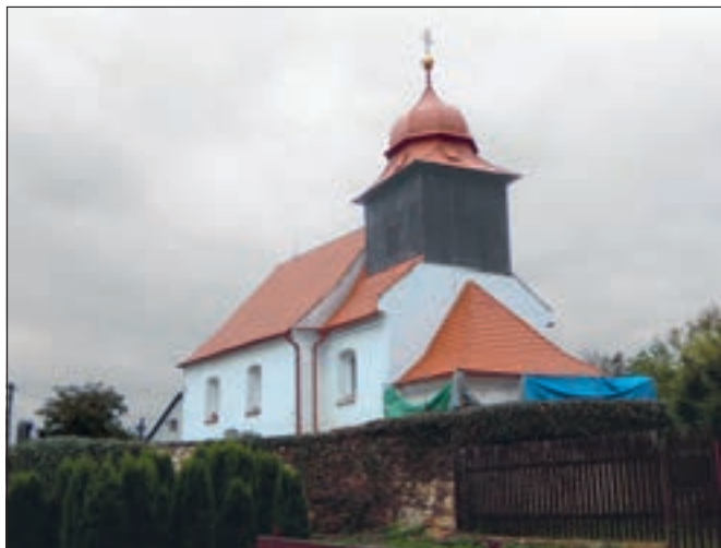
Tebov (okres Benešov), kostel sv. Prokopa, obnova střechy věže a sakristie. Krovová konstrukce byla v předešlém roce tesařsky opravena, protože byla poškozena zatékáním. V tomto roce byla bání plechována. Dále byla provedena obnova krovu a stropu nad sakristií a nevhodná plechová krytina byla nahrazena pálenými bobrovkami (foto D. Primusová).
