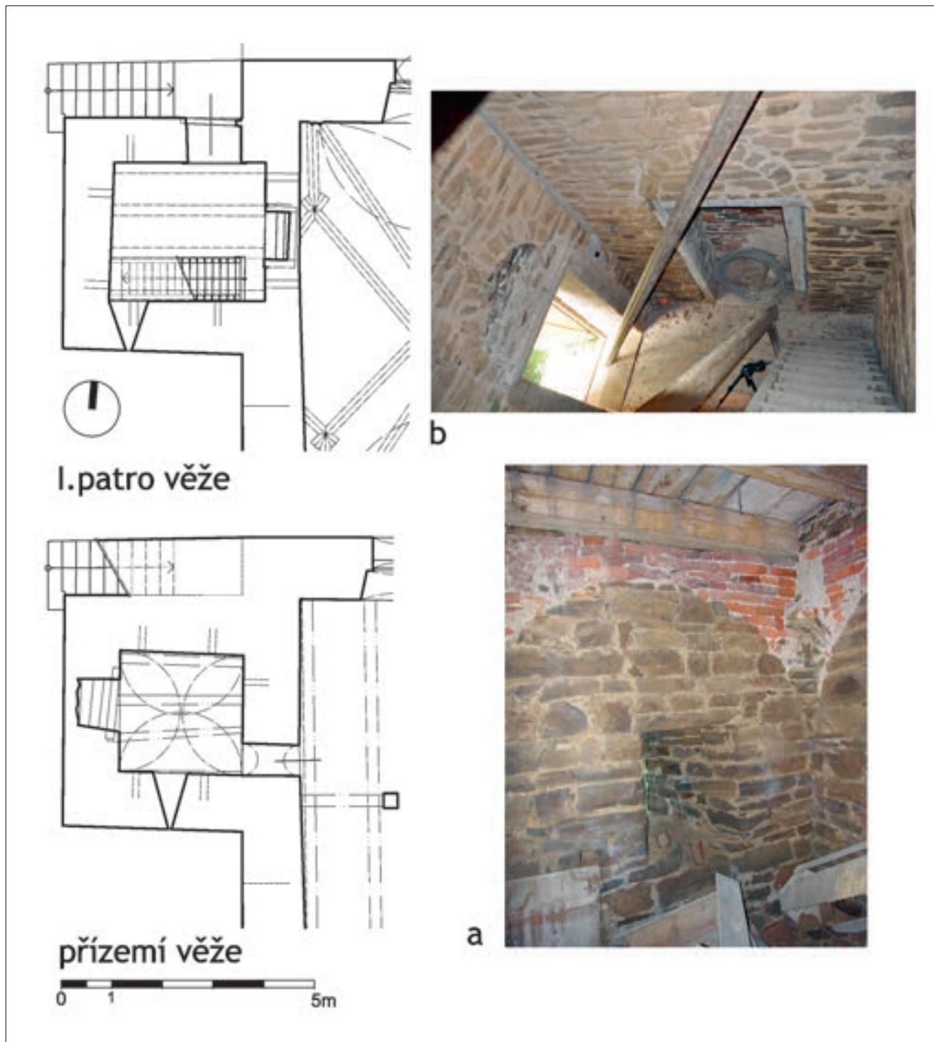
Neustupov (okres Benešov), kostel Nanebevzetí Panny Marie. V rámci probíhajícího stavebněhistorického průzkumu kostela je zpracováváno také zaměření současného stavu. K tomuto v jádře románského kostela totiž existoval doposud pouze jednoduchý půdorys v soupisu památek historických a uměleckých, který je pro potřeby SHP i projektové práce nepoužitelný. Nejintaktnější dochovanou částí románské stavby je západní věž: a – přízemí s torzem původní křížové klenby; b – patro s dvojicí románských portálů (zaměření J. Veselý a J. Kypta, kresba a foto J. Veselý).
