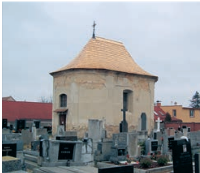
Rejštice (okres Mladá Boleslav), kaple sv. Jiljí po obnově střechy. V roce 2015 se podařilo opravit chátrající střechu kaple. Po důkladné opravě narušené krovové konstrukce byl položen štípaný šindel (foto D. Linhartová).
