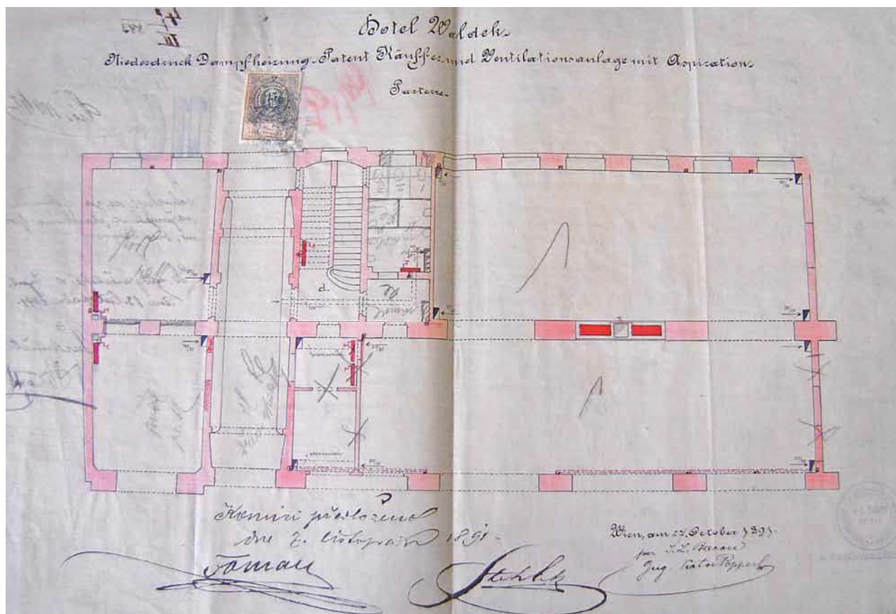
Obr. 5. Victor Popperl: Hotel Waldek, návrh parního topení a přívodu ventilace. Přízemí. Vídeň, 27. 10. 1891. Kolorovaný rys tuší na papíře. Plán přízemí podle stavu ještě před přestavbou. (Magistrát města Plzně, reprofoto D. Linhartová, 2011)
