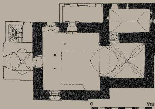
Půdorys kostela Neposkvrněného Početí Panny Marie
