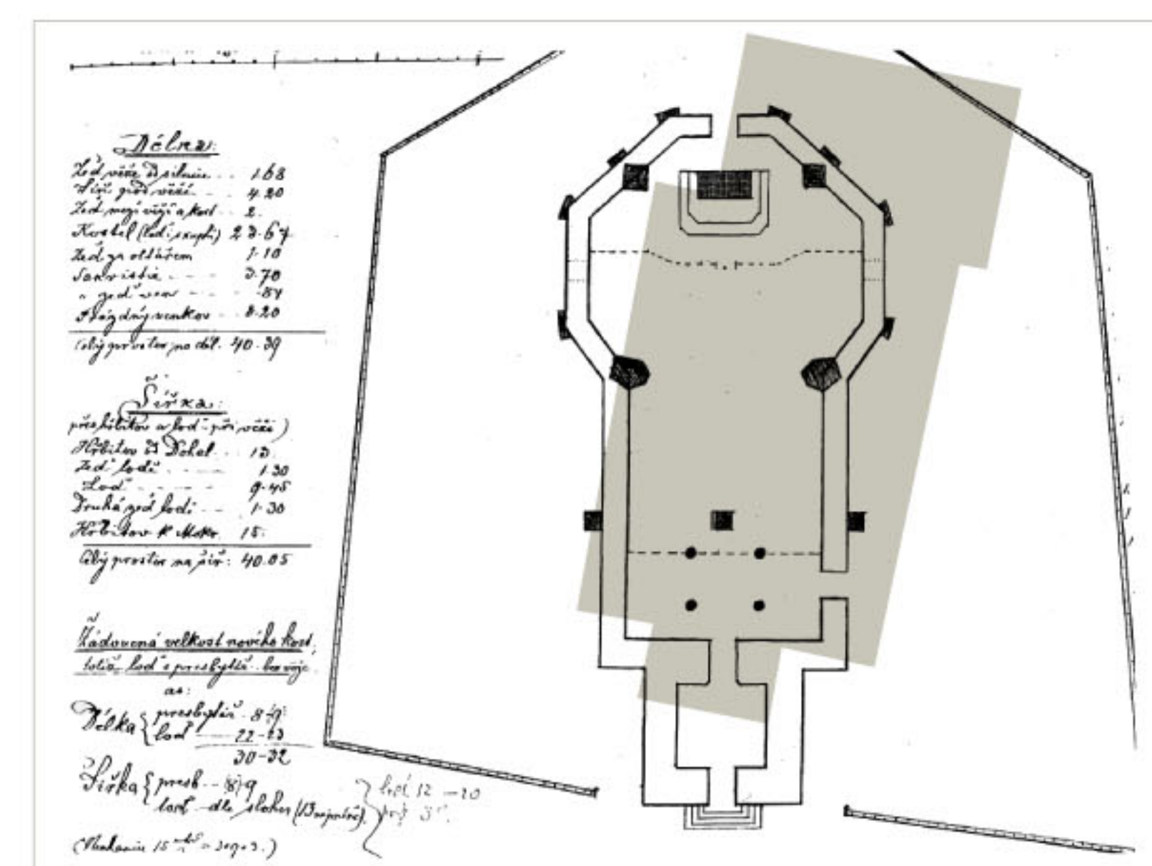
Půdorys kostela sv. Jana Křtitele ve stavu před zbořením v roce 1888. Barevná plocha představuje obrys současného kostela.
